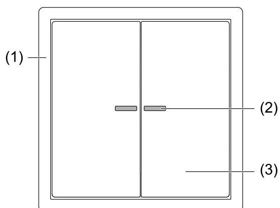
рисунок 2: Конструкция прибора, 2-местная
