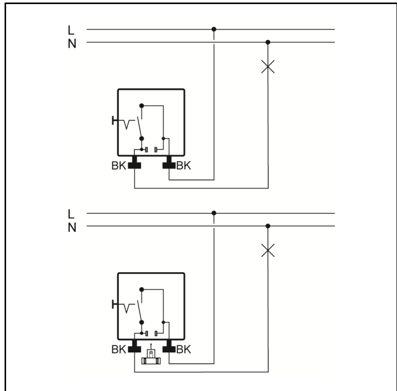
Wiring diagrams 501 U
